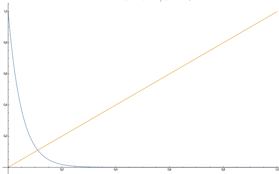
Рис. 4: x = e^{-\alpha x} , \alpha = 20
