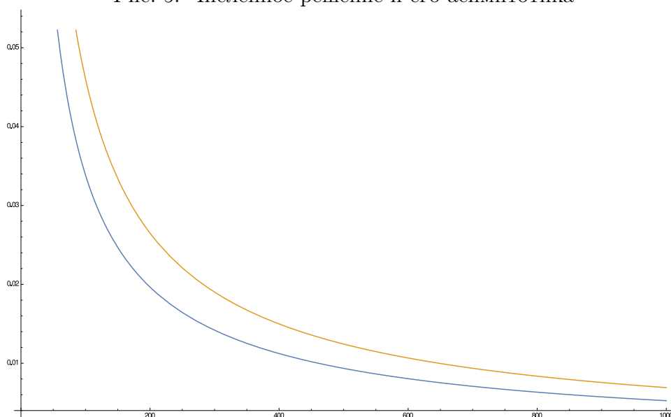
Рис. 5: Численное решение и его асимптотика
